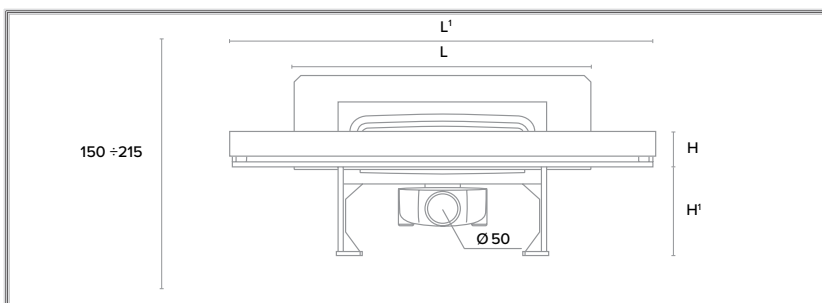
SIFONE DI SCARICO ribassato orientabile
